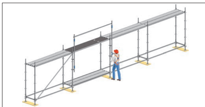
Fig. 37: Utilización de la barandilla de montaje en el modulo de acceso.
