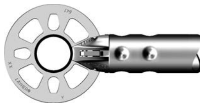
Fig. 3: Allround de aluminio según Z-8.22-64.1
