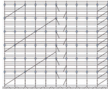
Fig. 94: Módulo de anclaje 4,00 m.
