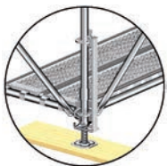
Fig. 82: Aseguramiento de base con cabeza con cuña
