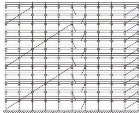
Fig. 95: Módulo de anclaje 2,00 m.
